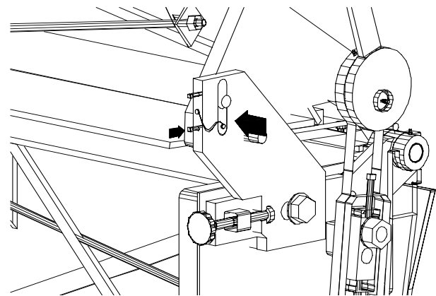
Soporte Especial Media-Luna cuando se dobla con Angulo Peinado (Fijar con Tornillo Inferior)
